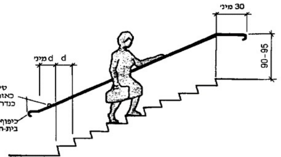
ציור 12 - חתך בית-אחזה במדרגות
