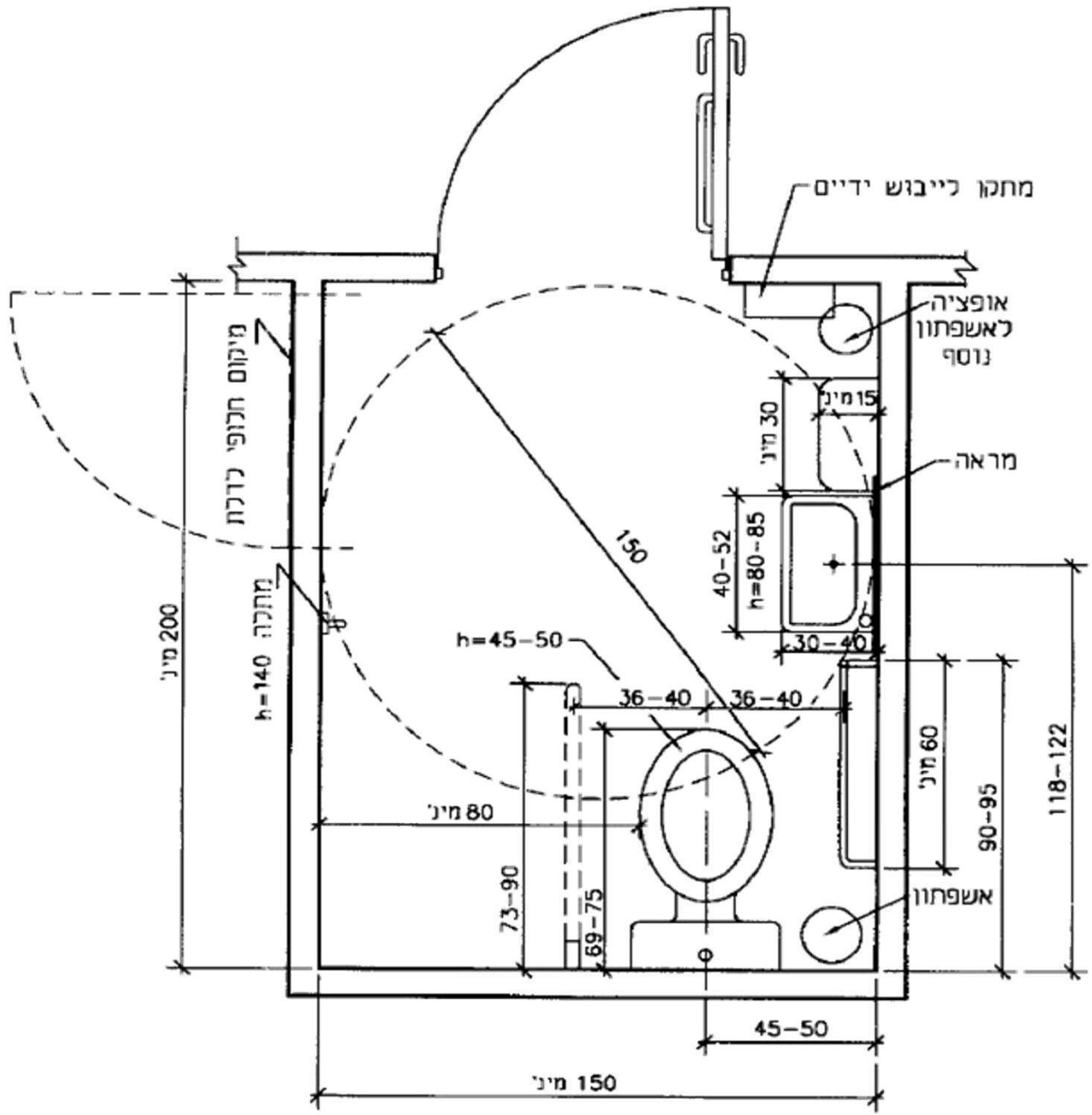
ציור 16 - תא שירותים עם אסלה פינתית (המידות בסנטימטרים)
