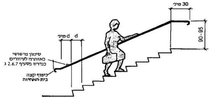
ציור 12 - חתך בית-אחיזה במדרגות
