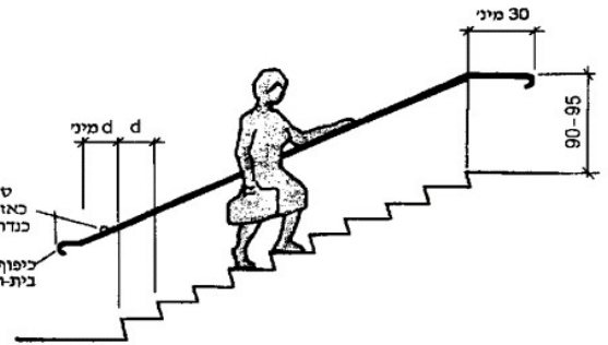
ציור 12 - חתך בית-אחיזה במדרגות
